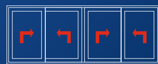
4-teiliges Element mit 4 Hebe-Schiebeflügeln
